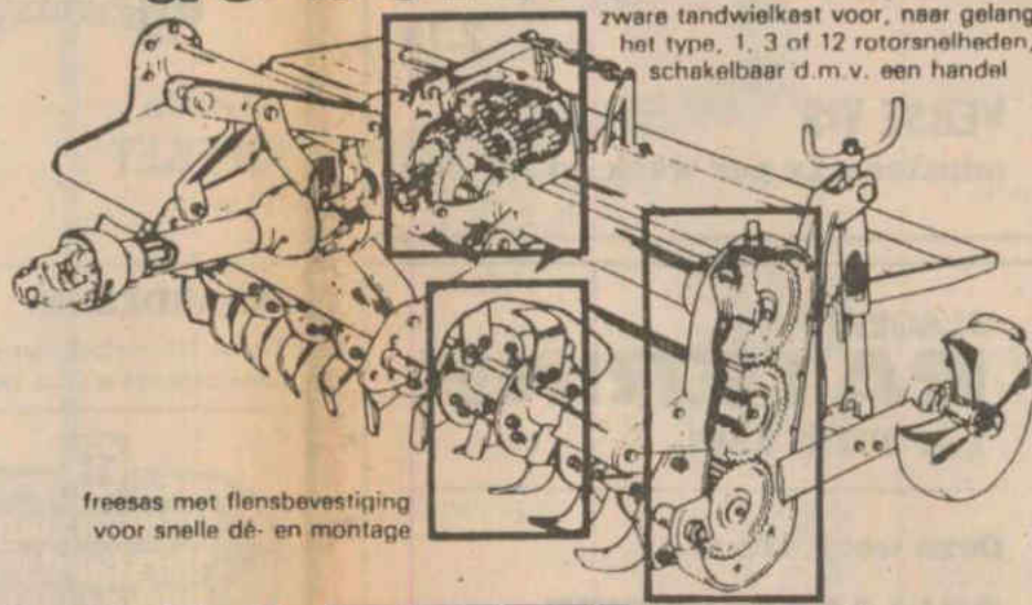
uiterst solide aandrijving d.m.v. tandwielen
